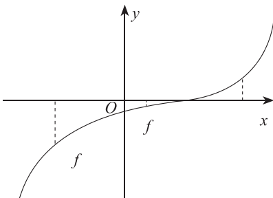
图5-3 二分法
