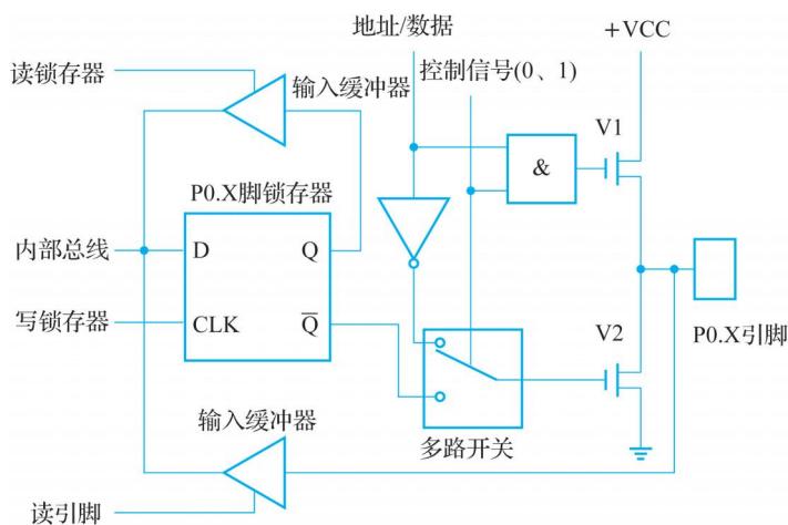
图 1-13 P0 口工作原理图
