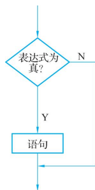
图 1-25 if 语句结构图
