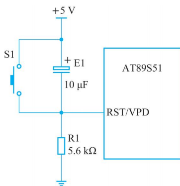
图 1-10 混合复位电路
