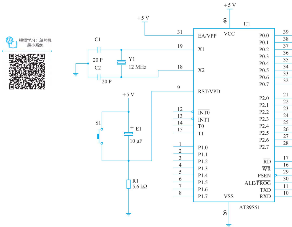
图 1-11 单片机最小系统电路图
