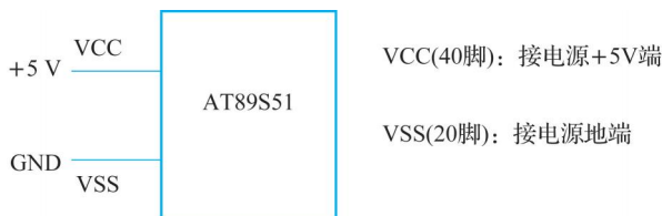
图 1-5 单片机电源原理图
