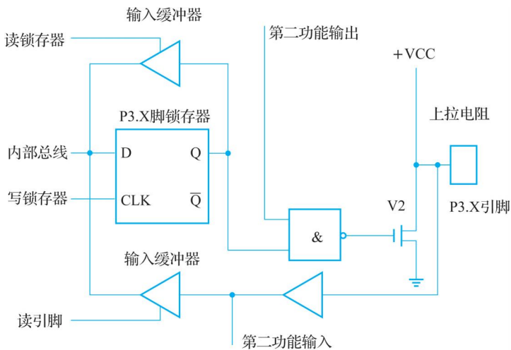
图 1-19 P3 口工作原理图
