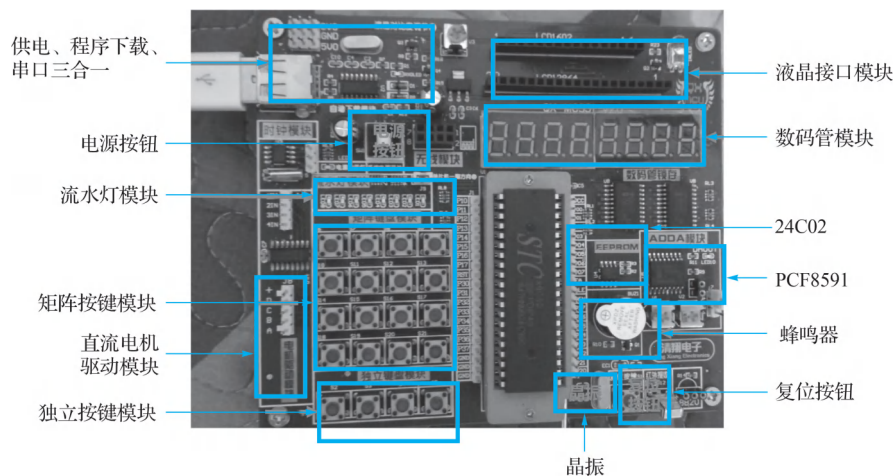
图 1-30 实验板结构图
