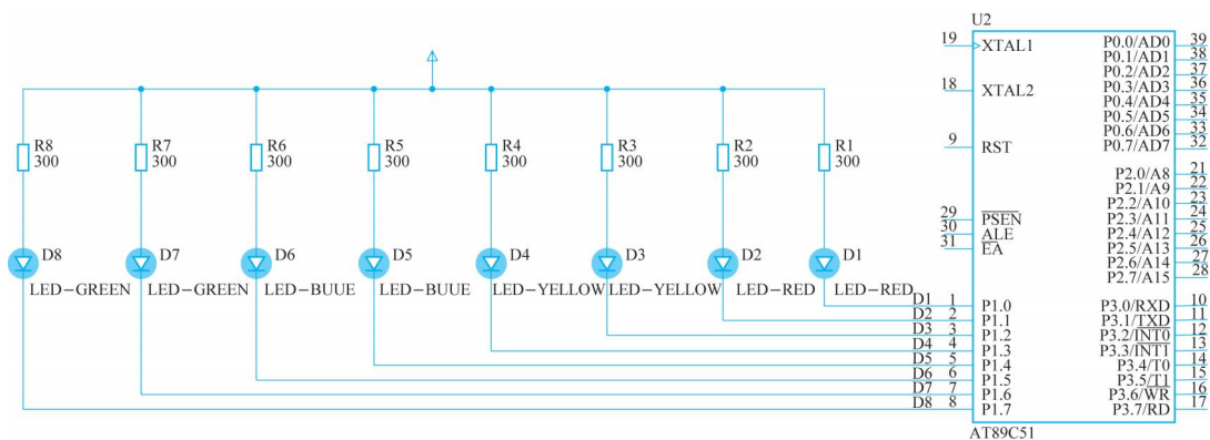
图 1-24 在 Proteus 中，单片机控制 LED 彩灯仿真图
