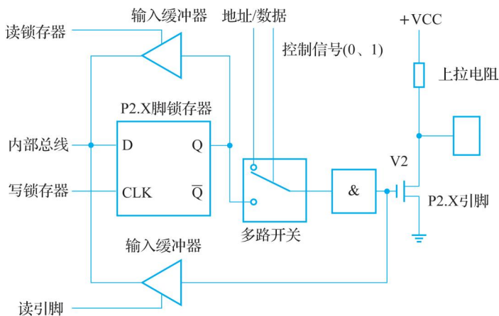
图 1-18 P2 口工作原理图
