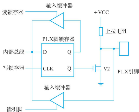
图 1-17 P1 口工作原理图
