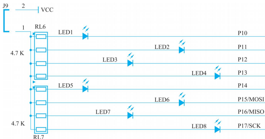
图 1-32 实验板彩灯电路原理图
