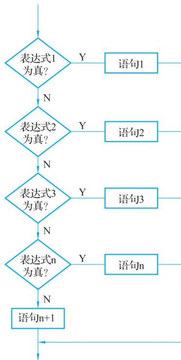
图 1-27 if-else—if 多分支结构图
