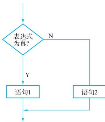
图 1-26 if-else 结构图
