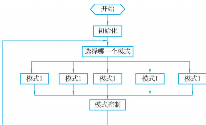
图 1-29 流程图样例
