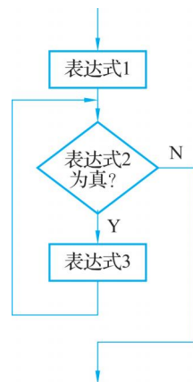
图 1-28 for 循环流程图
