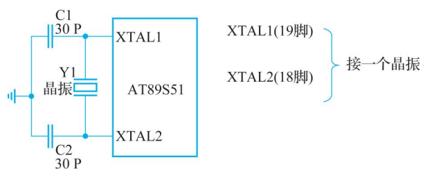
图 1-6 单片机时钟电路
