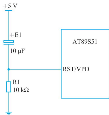
图 1-8 单片机上电复位电路
