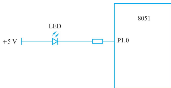
图 1-23 单片机控制 LED 灯原理图
