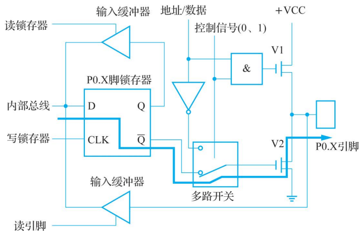
图 1-14 P0 口内部数据总线向引脚输出示意图
