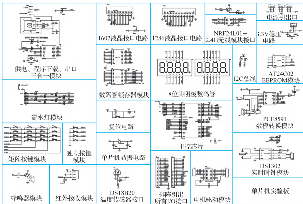
图 1-31 实验板原理图
