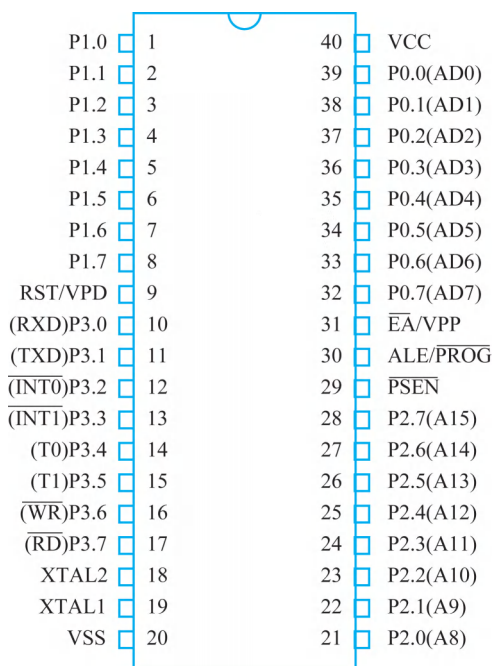
图 1-2 8051 系列单片机的引脚图
