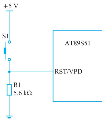
图 1-9 按键复位电路
