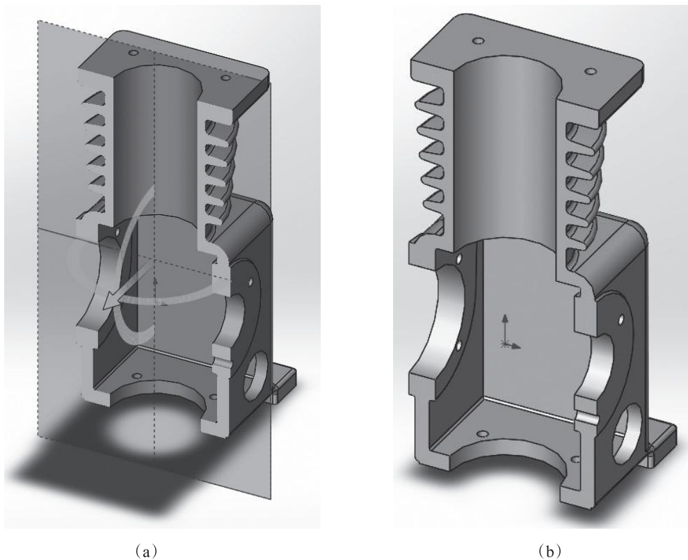
图 1-2-6 剖面图
