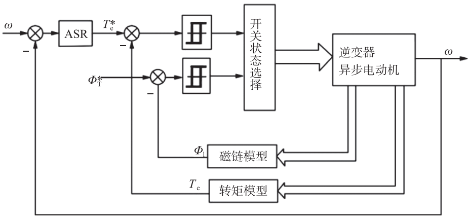
图 2-14 按定子磁场控制的直接转矩控制系统原理框图
