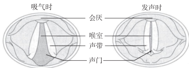
图 1-2 发声器官
