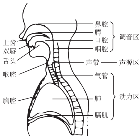
图 1-3 共鸣腔体
