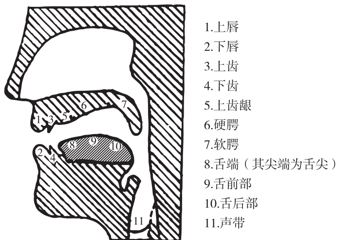
图 1-4 咬字器官
