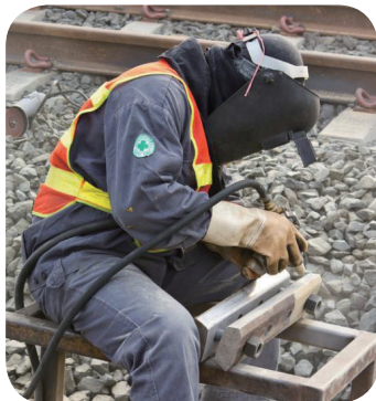
图 1-3 焊接
